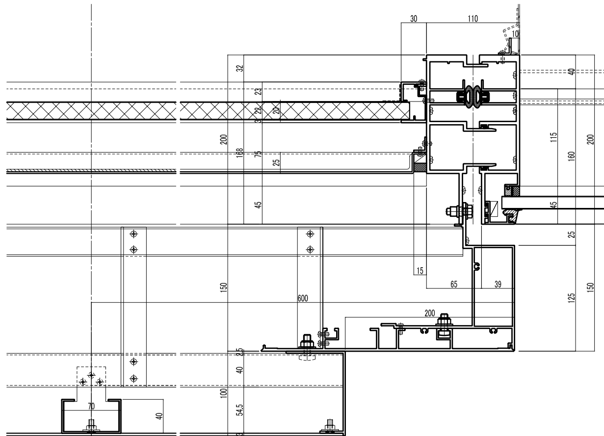
縦断面図
