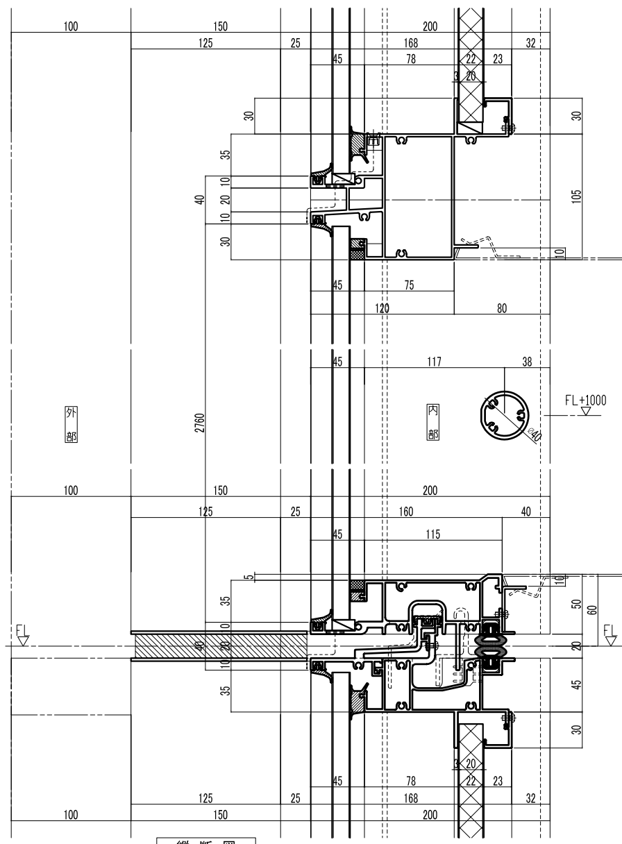
縦断面図
