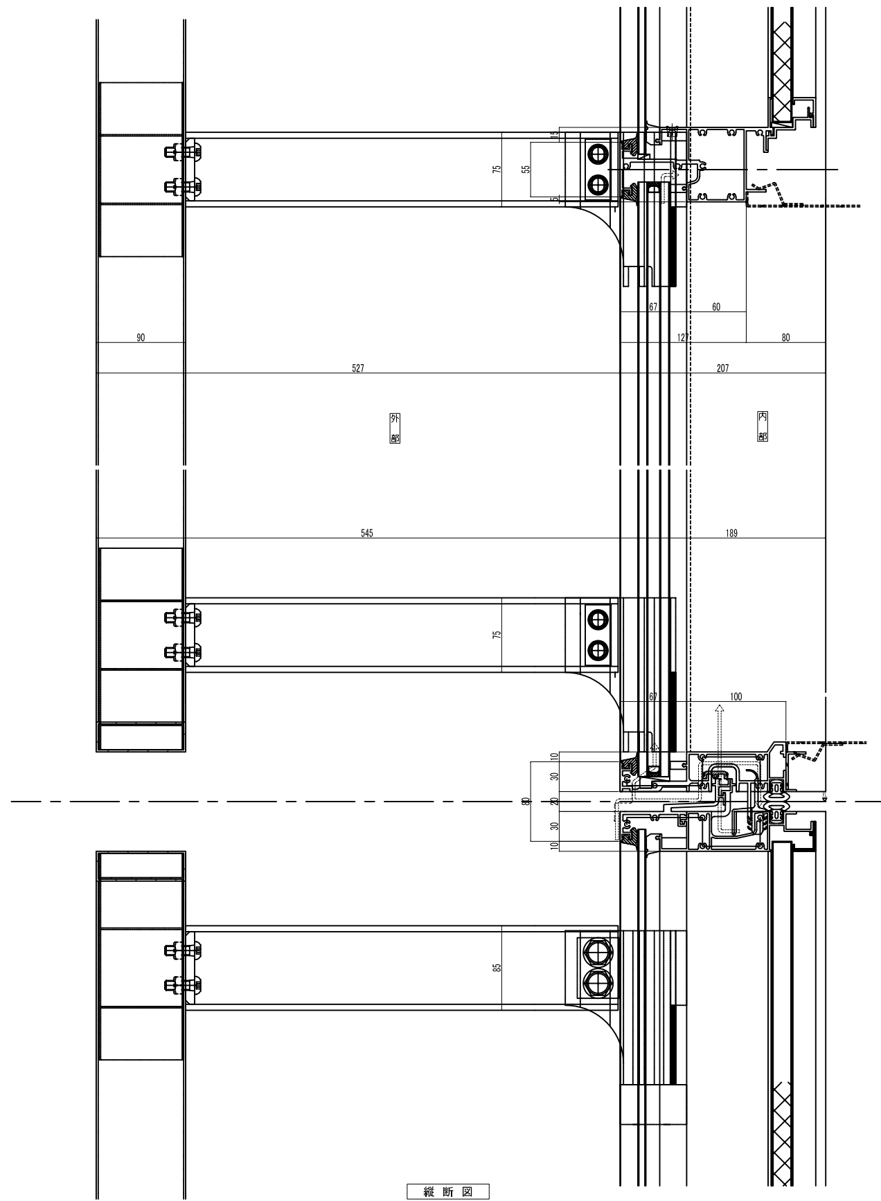
縦断図
