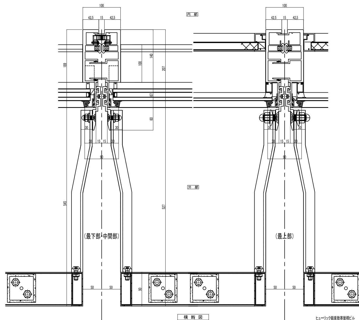
外観図
