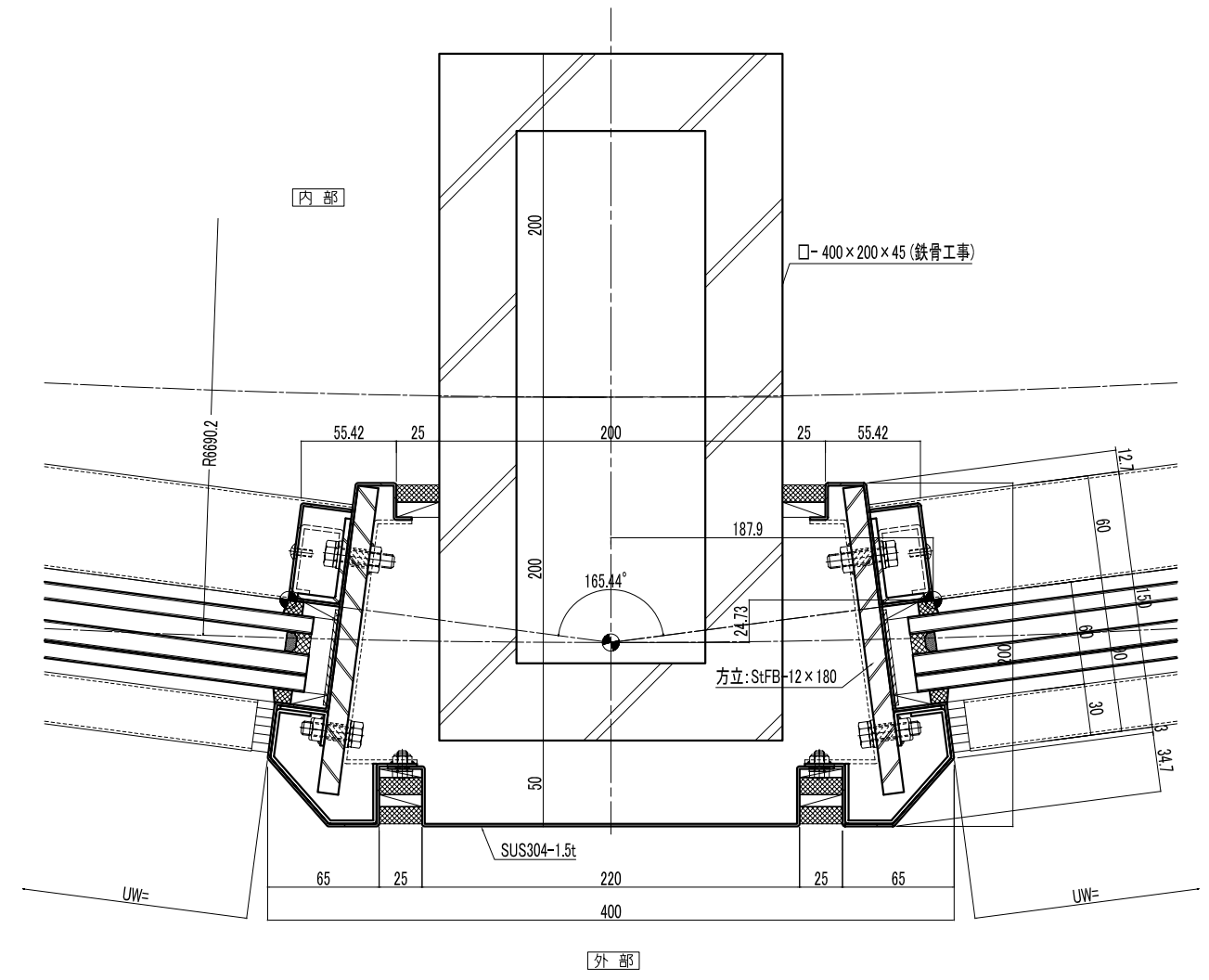
横断図 (5FL+150)
