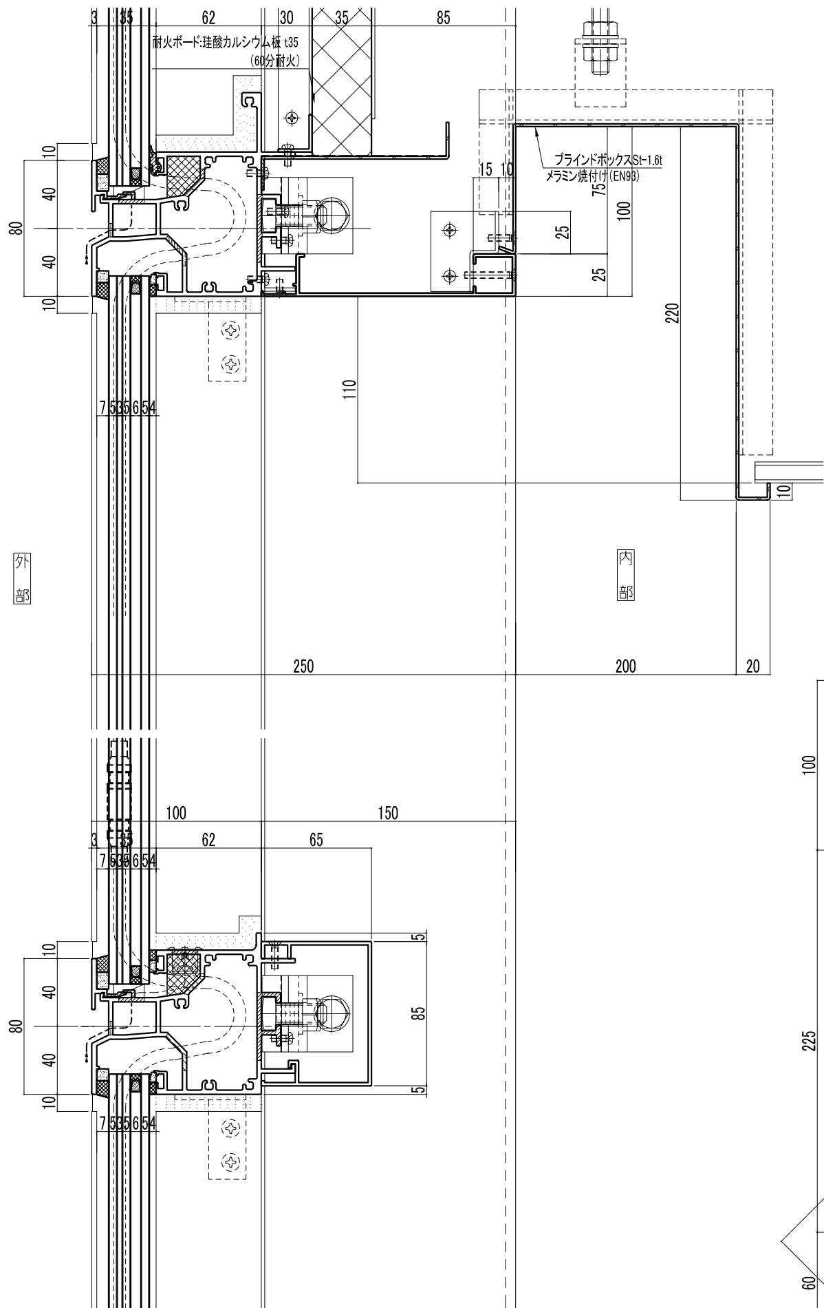
縦断図
