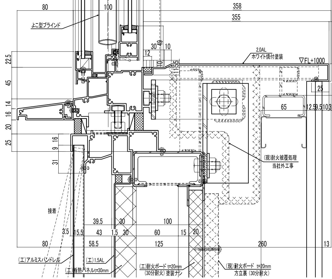
縦断図
