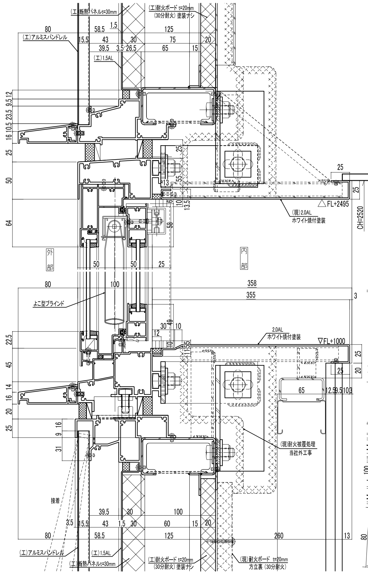
縦断図
