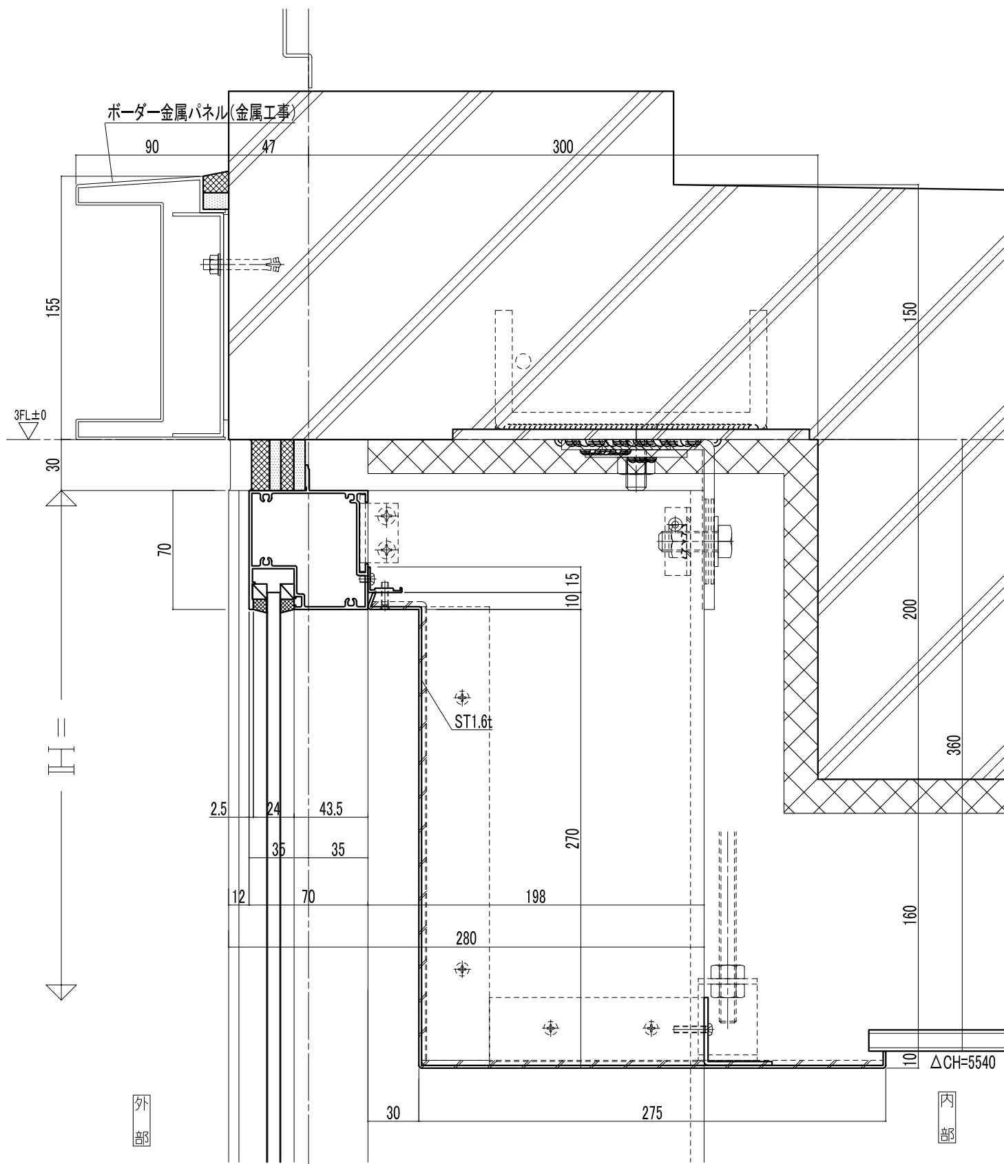
縦断図
