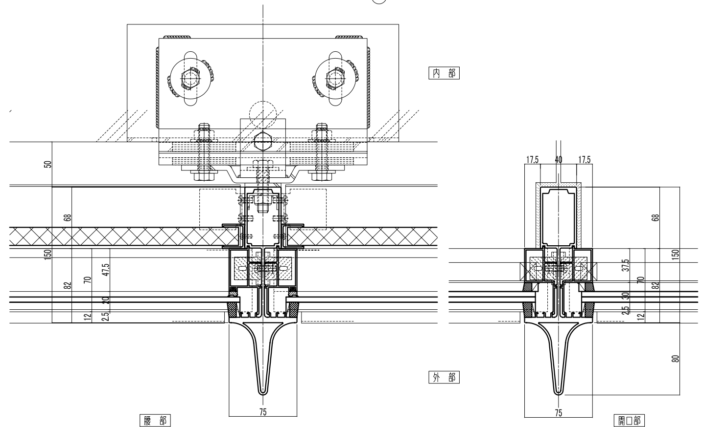
横断図
