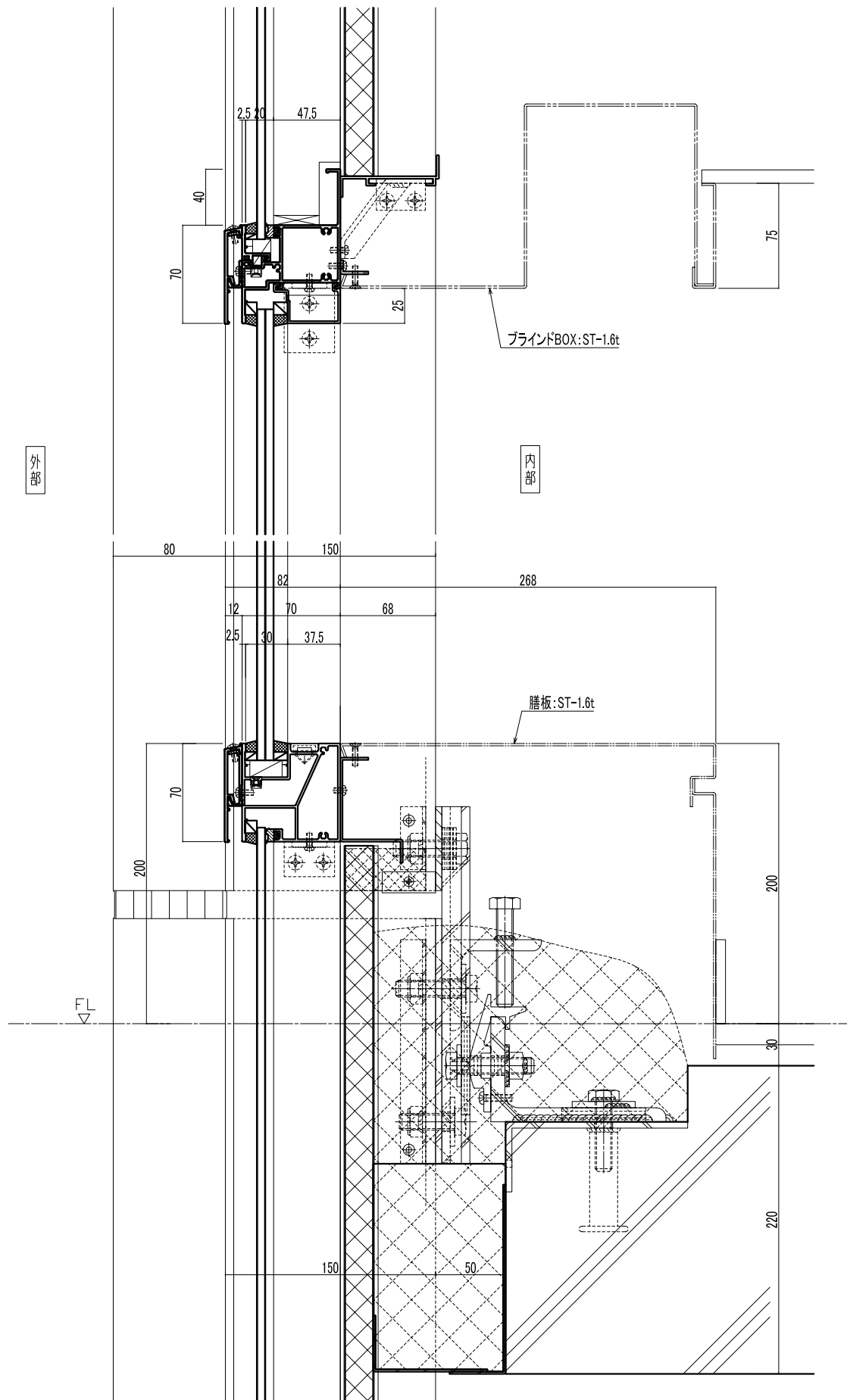
縦断図
