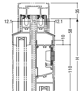
(ガラス溝幅 36mm)
